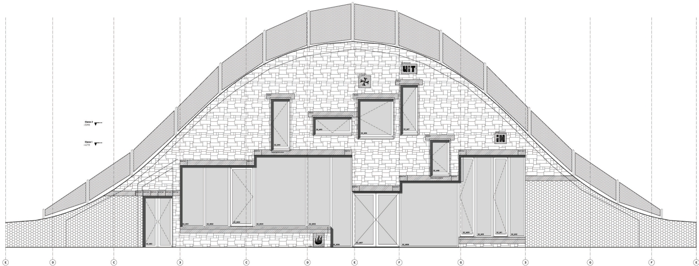
Abwicklung der Fassade entlang Ellipse
